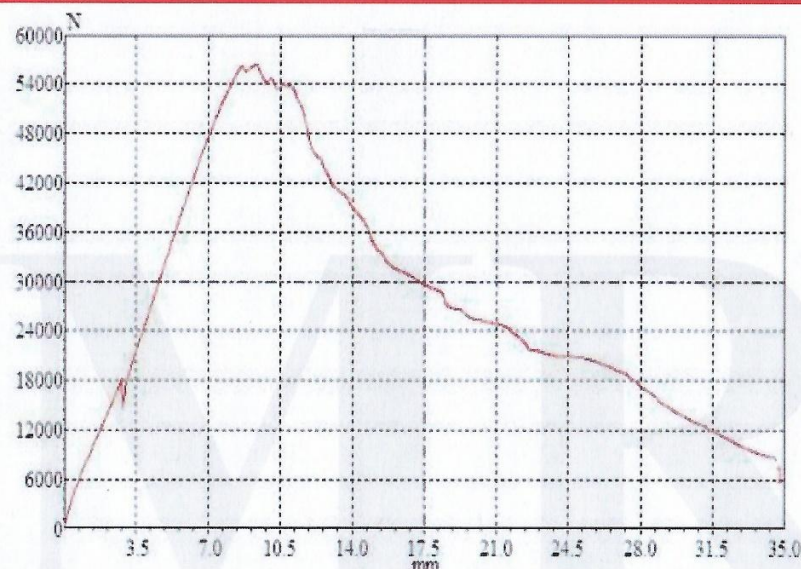
نمودار نیرو-جابجایی آزمون
